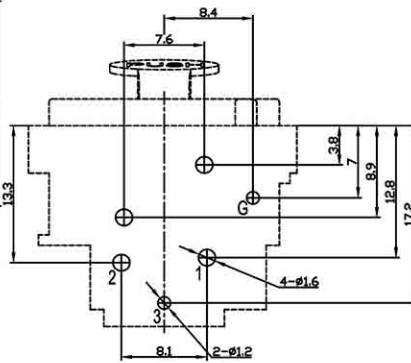
印制线路板示意图(底视图) PCB Layout(Bottom View)
